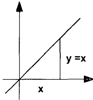
Figura 2: Curva que representa la función y = x . Para cada valor de x , el valor de y es el mismo.
