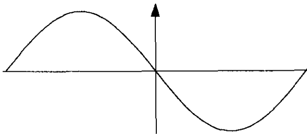
Figura 6: Curva que representa la función y = \text{sen}(x) . Conforme avanzamos y avanzamos en el eje x , los valores de y se van repitiendo en forma periódica.
