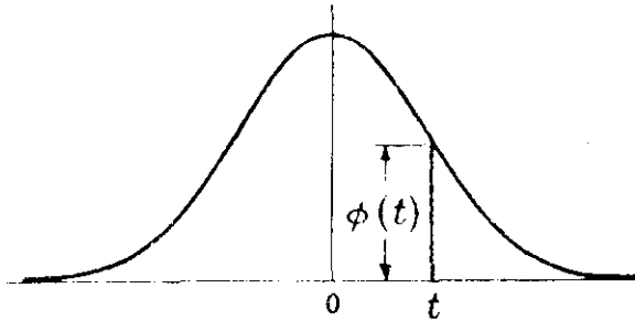
Figura 8: Curva que representa la función y = ce^{-kx^2} . El valor más alto de la "campana" lo alcanza en el punto conocido como la media de los valores de x (En nuestra figura, la media \mu está localizada en el cero).
